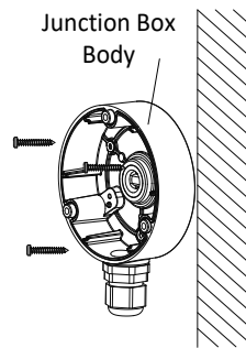
Рис. 2-6 Установка монтажной коробки на потолке / стене
