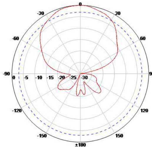
Вертикальная, 3 дБ
