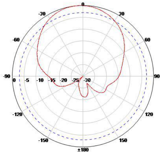
Горизонтальная, 3 дБ
