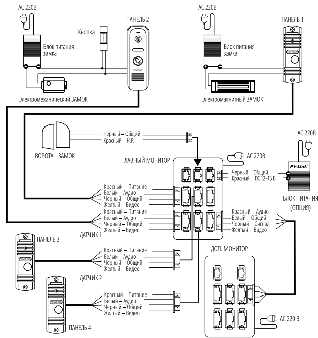
Рис. 8 Схема подключения видеодомофонов MAGIC 7 HD ver.4821|4822
