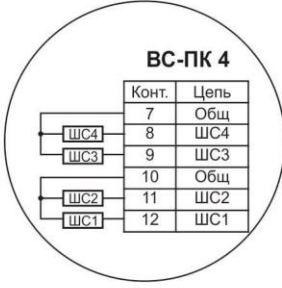
Рис.2. Схемы внешних соединений приборов:
