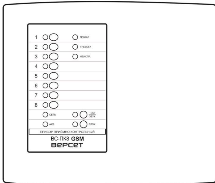
Рис.1. Внешний вид передней панели приборов BC-ПК2 GSM версия 2.2, BC-ПК4 GSM версия 2.2, BC-ПК8 GSM версия 2.2.
