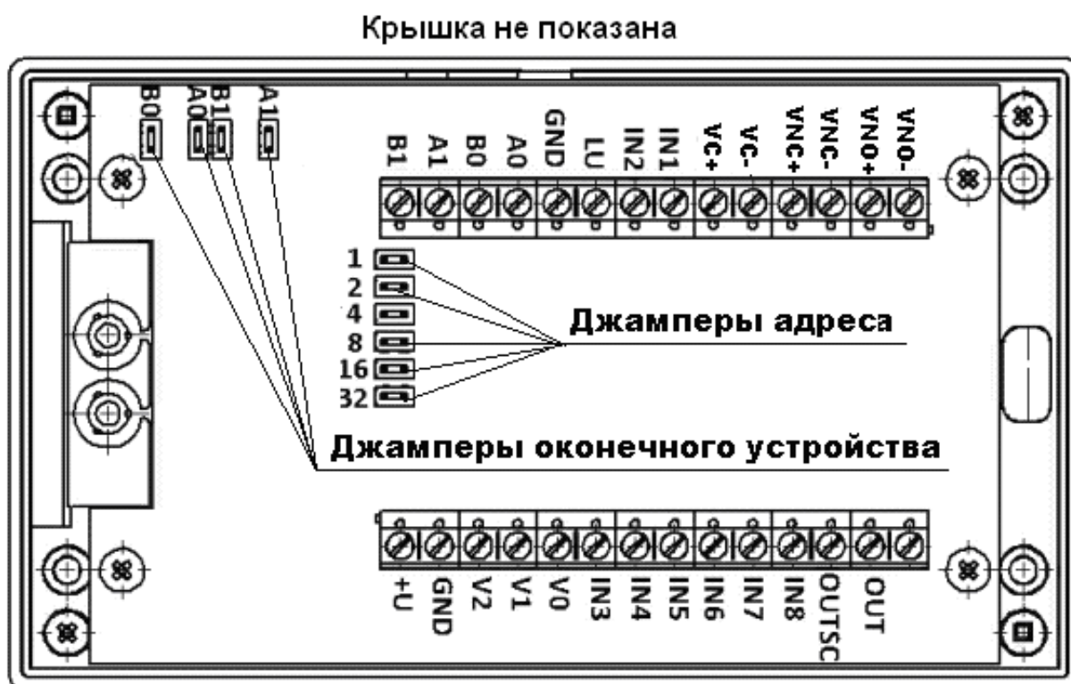
Рис.2 Вид КМ500-8.3Т со снятой крышкой.
