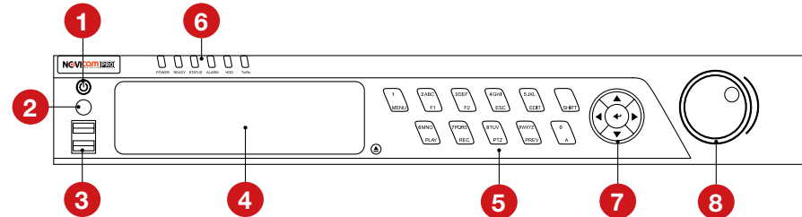
Рисунок 3.5 Передняя панель IP регистраторов (корпус под 4 HDD).
