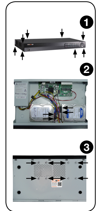
Рисунок 3.2 Установка HDD в IP регистраторах.
