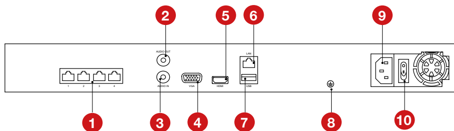
Рисунок 3.7 Задняя панель IP регистраторов (корпус под 2 HDD, 4 PoE).
