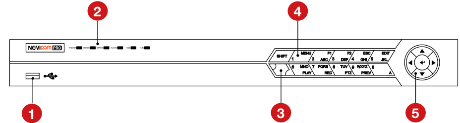
Рисунок 3.4 Передняя панель IP регистраторов (корпус под 2 HDD).
