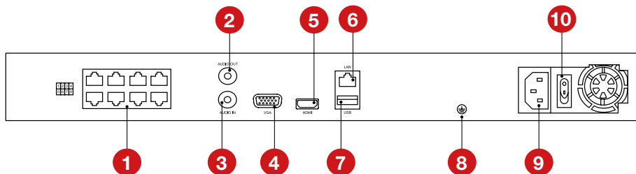
Рисунок 3.9 Задняя панель IP регистраторов (корпус под 2 HDD, 8 PoE).
