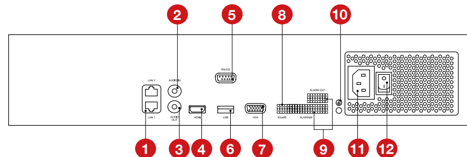
Рисунок 3.10 Задняя панель IP регистраторов (корпус под 4 HDD).
