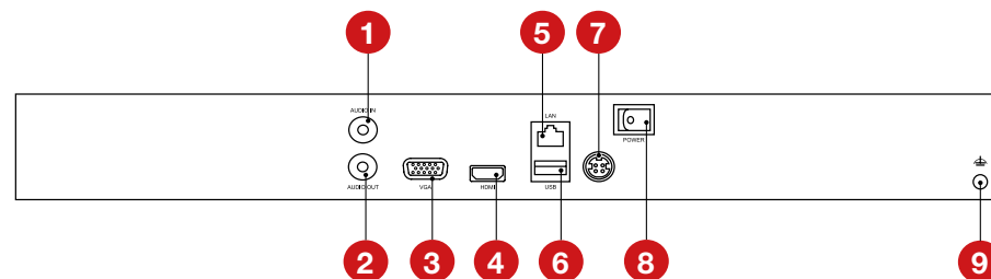
Рисунок 3.8 Задняя панель IP регистраторов (корпус под 2 HDD).
