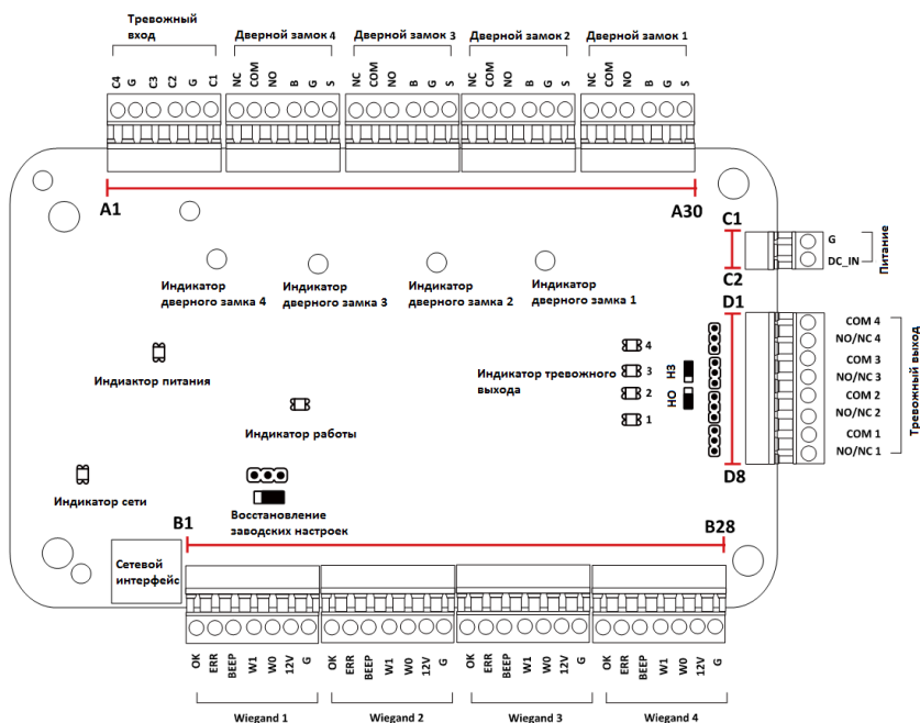
Рисунок 3-3 Клеммы DS-K2804
