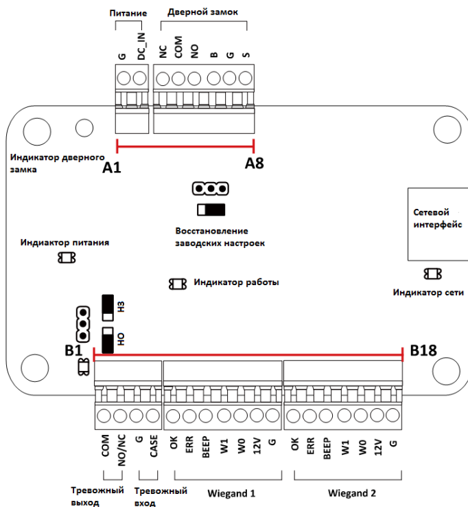
Рисунок 3-1 Клеммы DS-K2801
