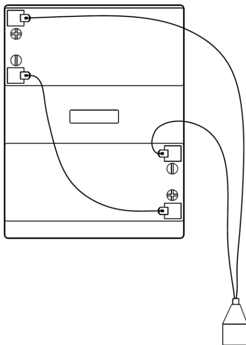
Рисунок 7 — схема соединений АКБ
