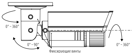
Рис. 10 Регулировка угла обзора видеокамеры Н1Т ×8
