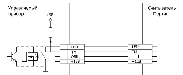
Рисунок 2 – Схема подключения считывателя к управляемому прибору
