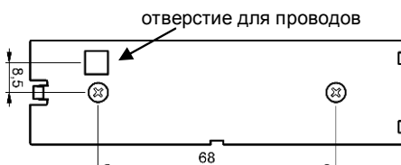
Рисунок 1 – Разметка для крепления к стене
