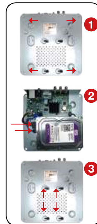
Рисунок 3.1 Установка HDD в аналоговых регистраторах.
