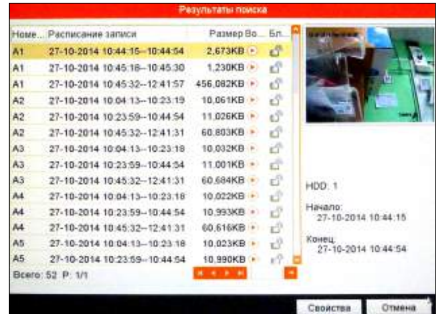
Рисунок 5.21 Результаты поиска.
