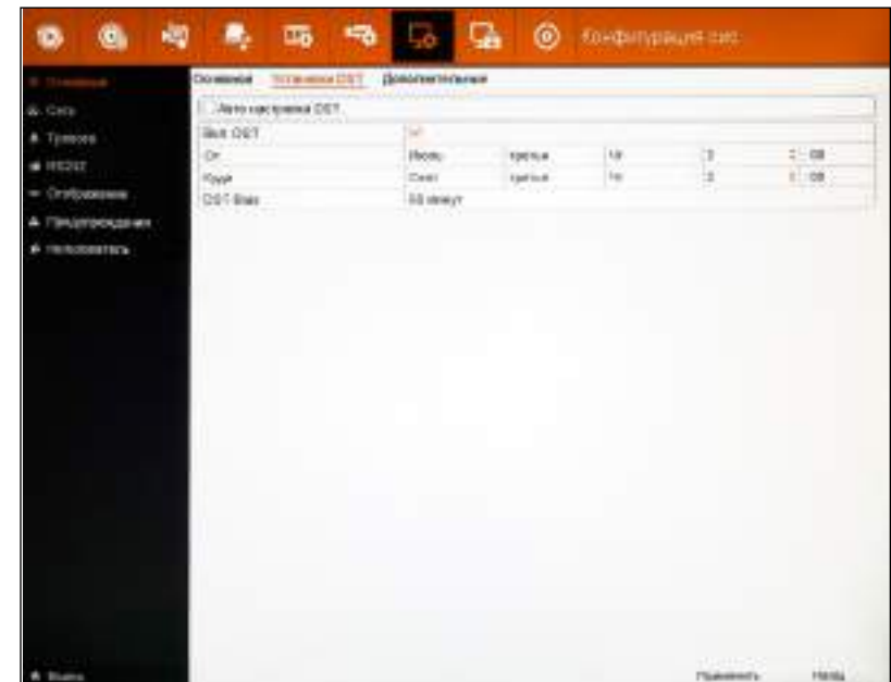
Рисунок 5.67 Установки DST.
