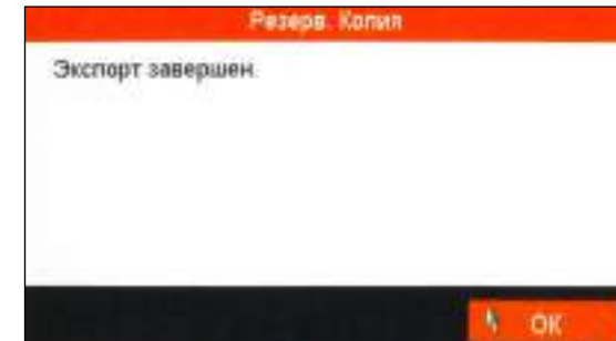
Рисунок 5.23 Экспорт завершён.
