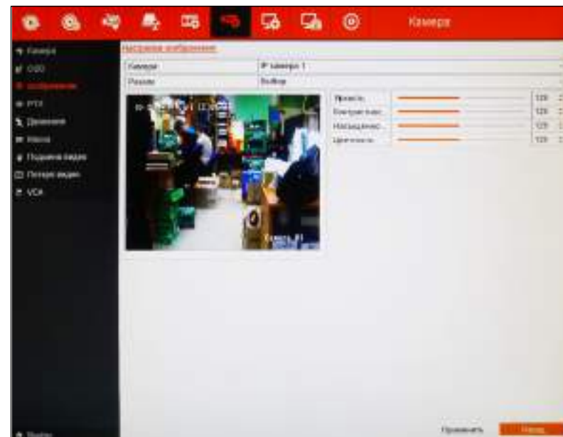
Рисунок 5.50 Настройка изображения.
