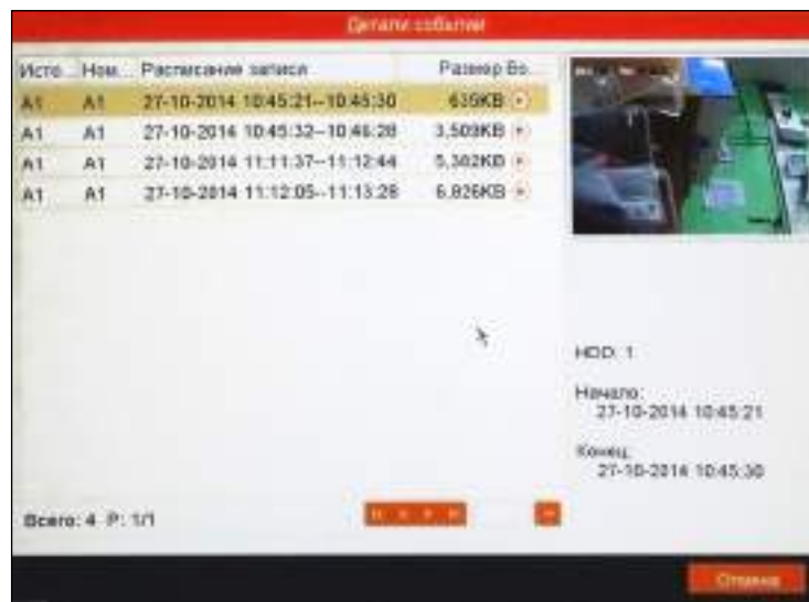
Рисунок 5.11 Детали.
