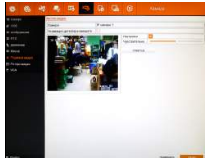
Рисунок 5.59 Заккрытие камеры.
