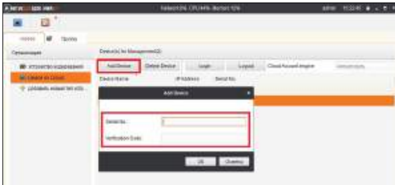
Рисунок 6.13 Добавление устройства.
