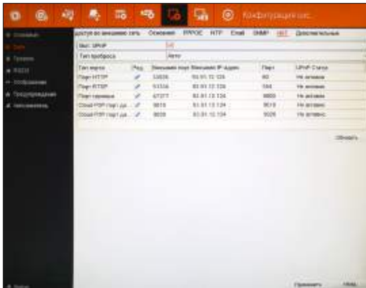
Рисунок 5.74 Настройка UPnP.
