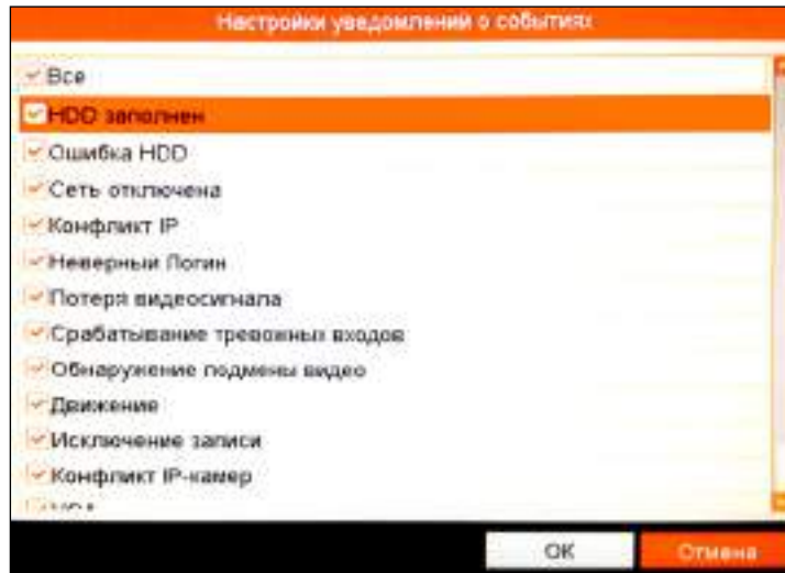
Рисунок 5.90 Подсказки событий.
