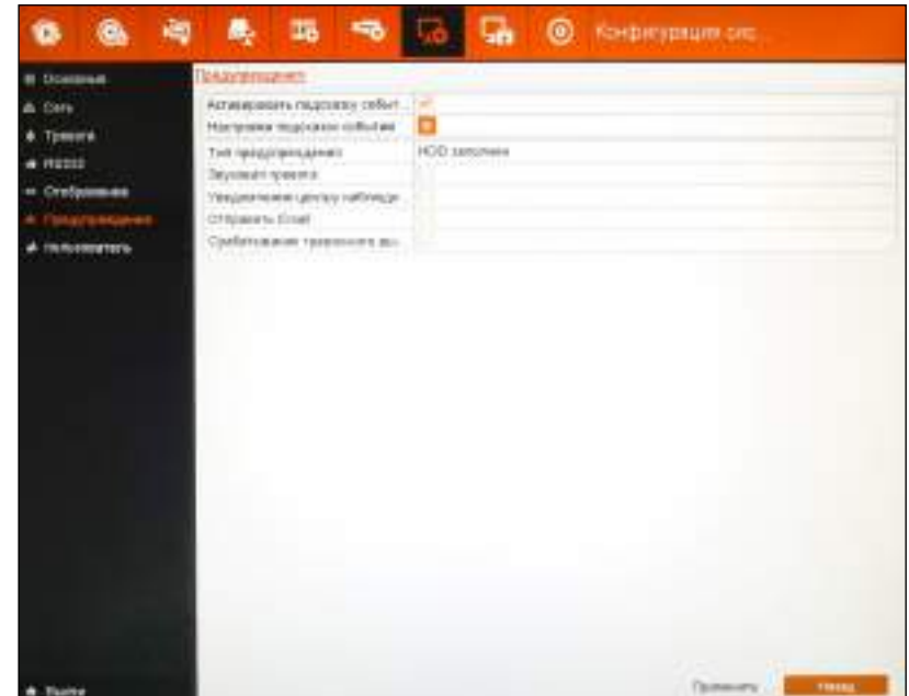
Рисунок 5.91 Предупреждения.
