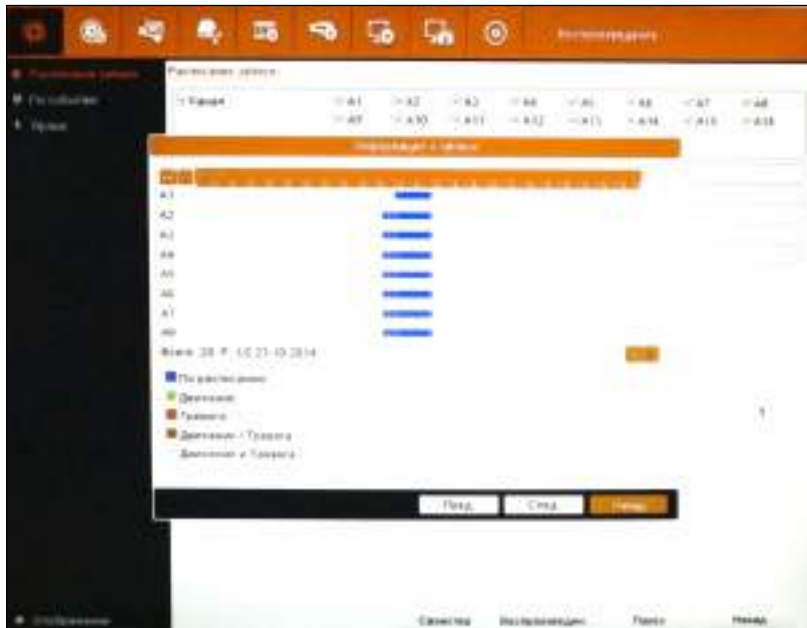
Рисунок 5.2 Свойства.
