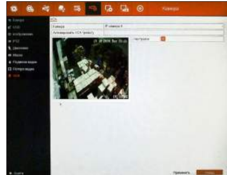
Рисунок 5.63 Видеоаналитика VCA.
