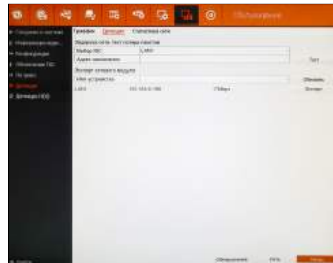
Рисунок 5.108 Детекция сети.
