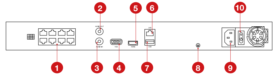
Рисунок 3.14 Задняя панель IP регистраторов (корпус под 2 HDD, 8 PoE).
