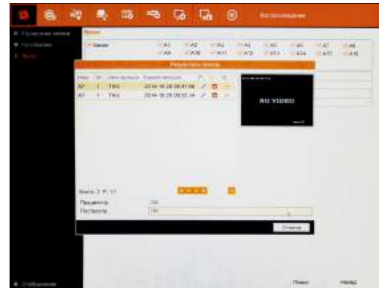
Рисунок 5.10 Найденные события.
