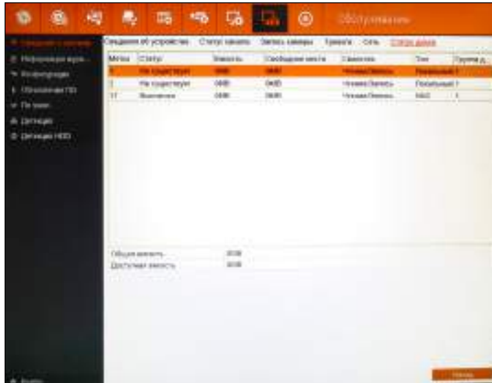
Рисунок 5.100 Статус диска.
