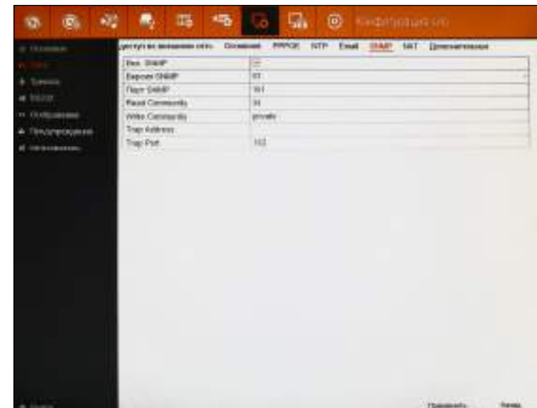
Рисунок 5.77 Настройка SNMP.
