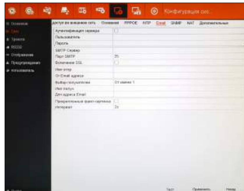
Рисунок 5.73 Настройка Email.
