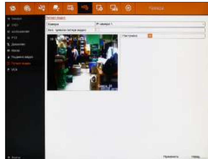
Рисунок 5.61 Потеря видео.
