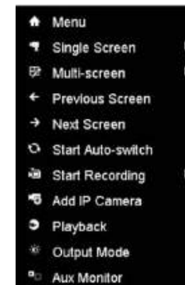
Рисунок 4.9 Всплывающее меню.
