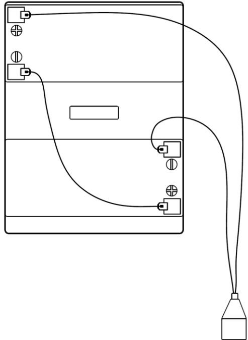
Рисунок 10 — Схема соединений АКБ в группе
