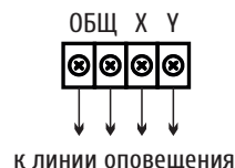
Рисунок 1. Схема подключения
