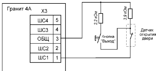
Рис. 7 Подключение цепей управления доступом
