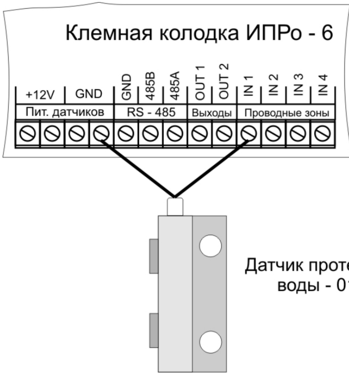
Подключение 1 датчика
