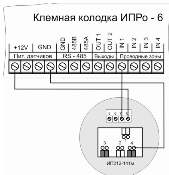
Подключение 1 датчика
