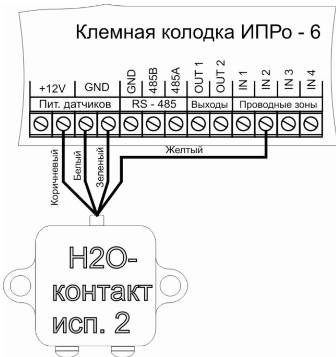
Подключение 1 датчика
