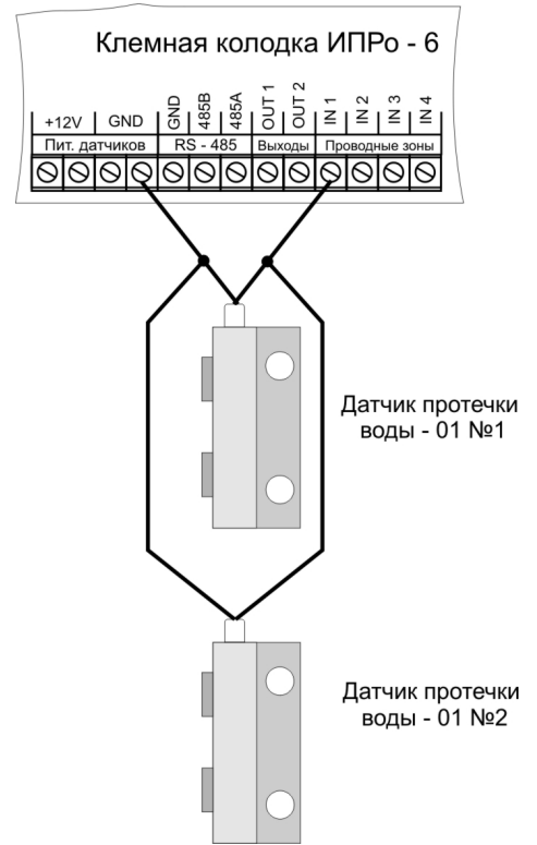
Подключение 2-х датчиков
