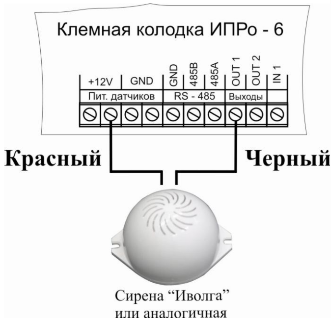
Подключение сирены с током потребления до 1А
