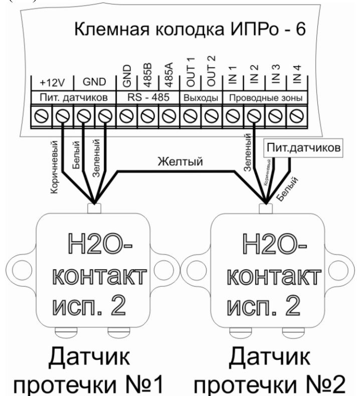
Подключение 2-х датчиков
