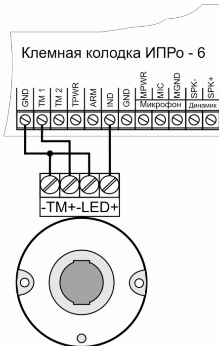
Считыватель ТМ
