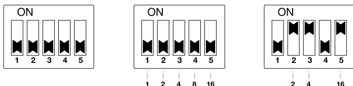
Рисунок 9. Пример установки адреса 22
