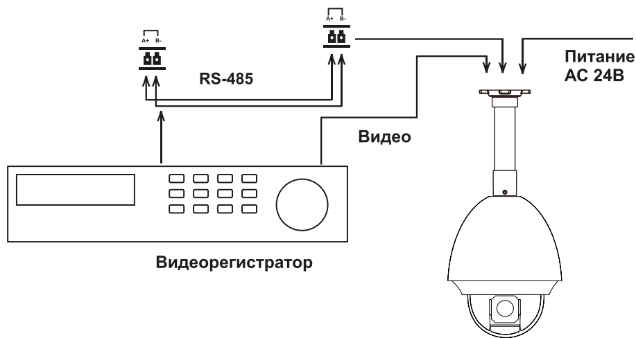
Рисунок 13. Подключение поворотной камеры к видеорегистратору с использованием RS-485.
