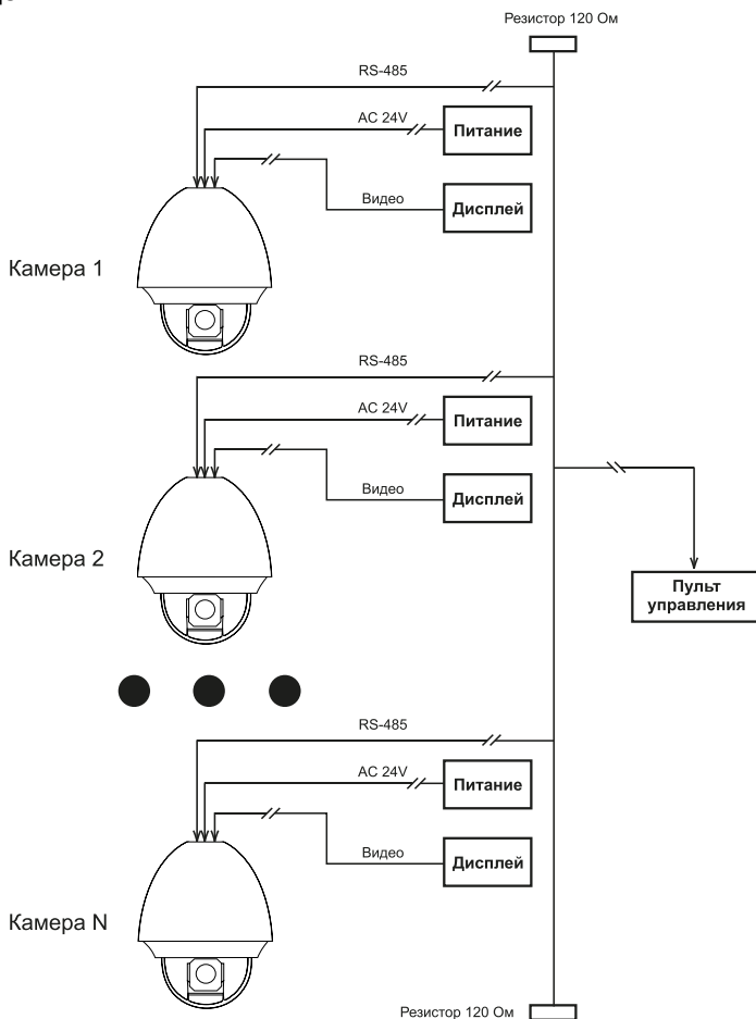
Рисунок 14. Подключение нескольких камер.
