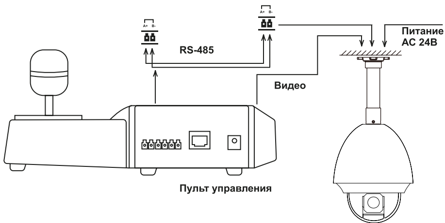
Рисунок 12. Подключение поворотной камеры к пульту управления/видеорегистратору.
