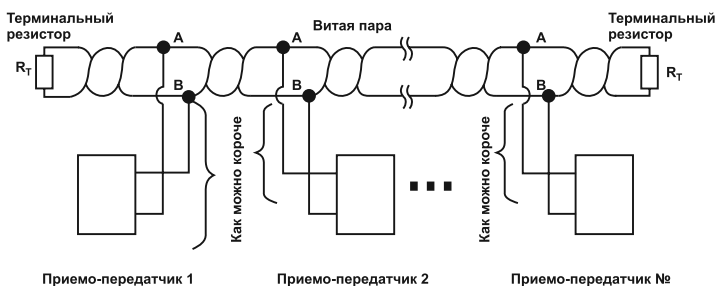
Рисунок 41. Схема подключения по RS-485.
