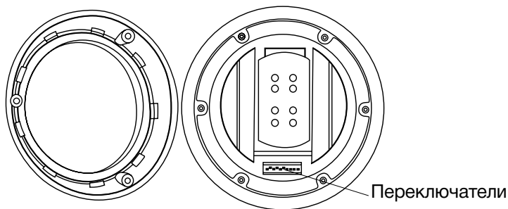
Рисунок 8. Расположение переключателей установки адреса и протокола.
