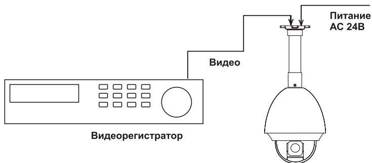
Рисунок 15. Подключение поворотной камеры к видеорегистратору.
