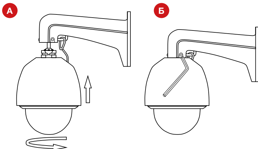
Рисунок 10. Установка скоростного купола.
