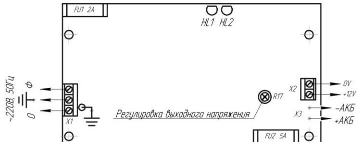
Схема подключения.
