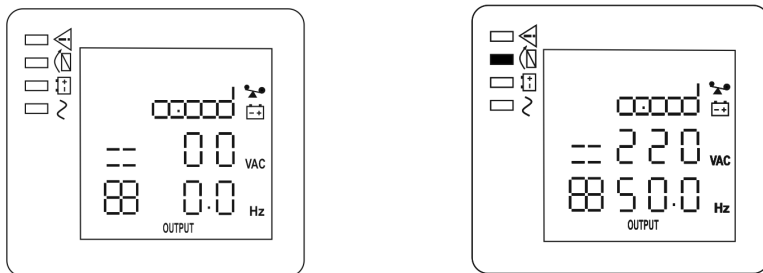
Рисунок 7 — состояние ЖК-дисплея при выключенном изделии и поданном на его вход сетевом напряжении
