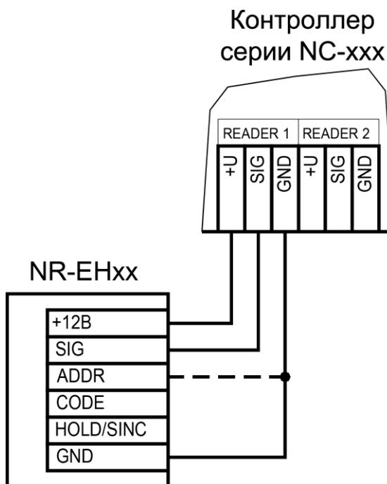
Рисунок 7. Адрес 1 (внутренний) – провод ADDR не подключен; адрес 0 (наружный) – провод ADDR подключен
