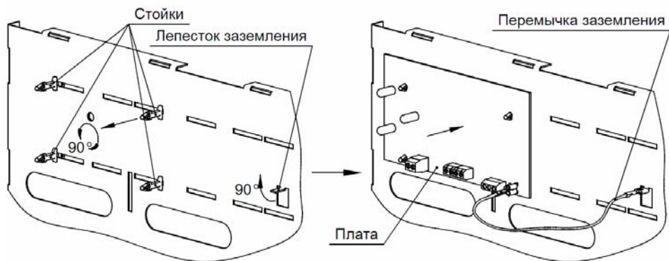
Рисунок 4. Установка платы
