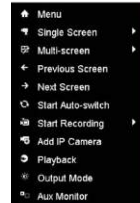
Рисунок 4.9 Всплывающее меню.
