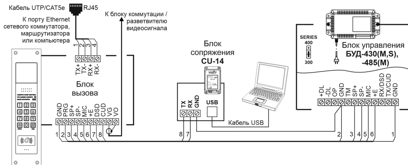
Рисунок 16.1 - Схема соединений блока вызова с блоками управления БУД-430(С, М), -485(М) и блоком сопряжения CU-14
