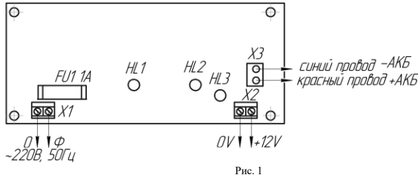
Схема подключения «ИВЭПР – 1230СП», «ИВЭПР – 1220СП»
