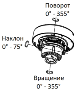
Рисунок 2.15 3-х осевая регулировка объектива
