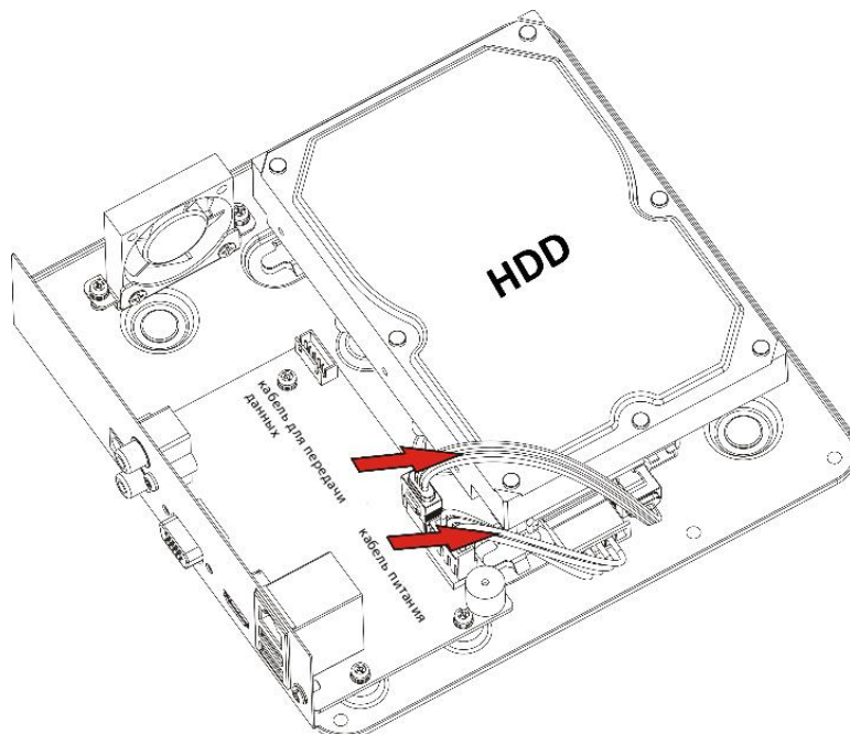
Рисунок 2.3 Подключение кабелей
