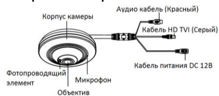
Рисунок 1-28 Панорамная камера
