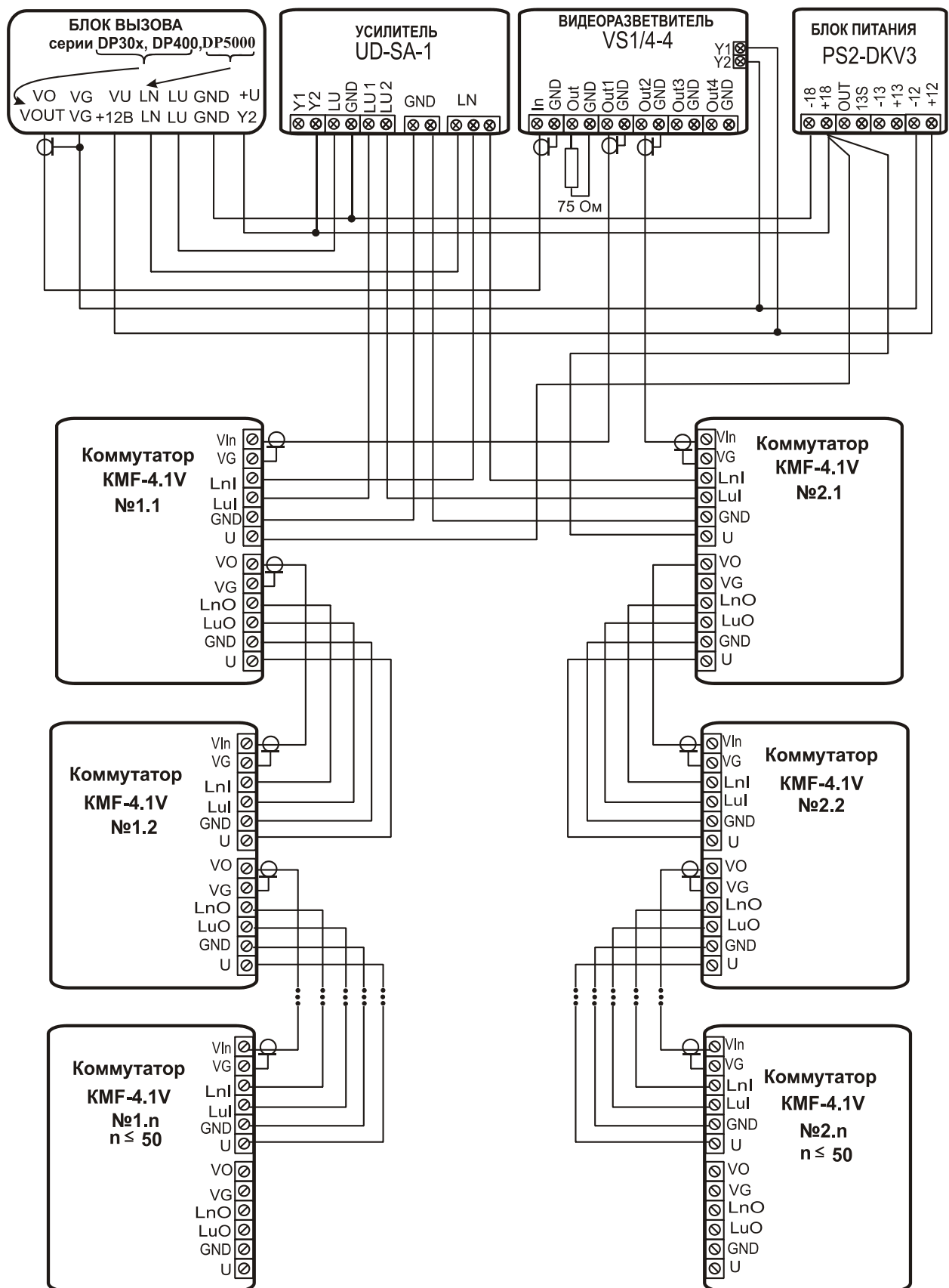
Рис.4 Схема подключения 100 (макс.) коммутаторов КМ- 4.1V по каналу управления
