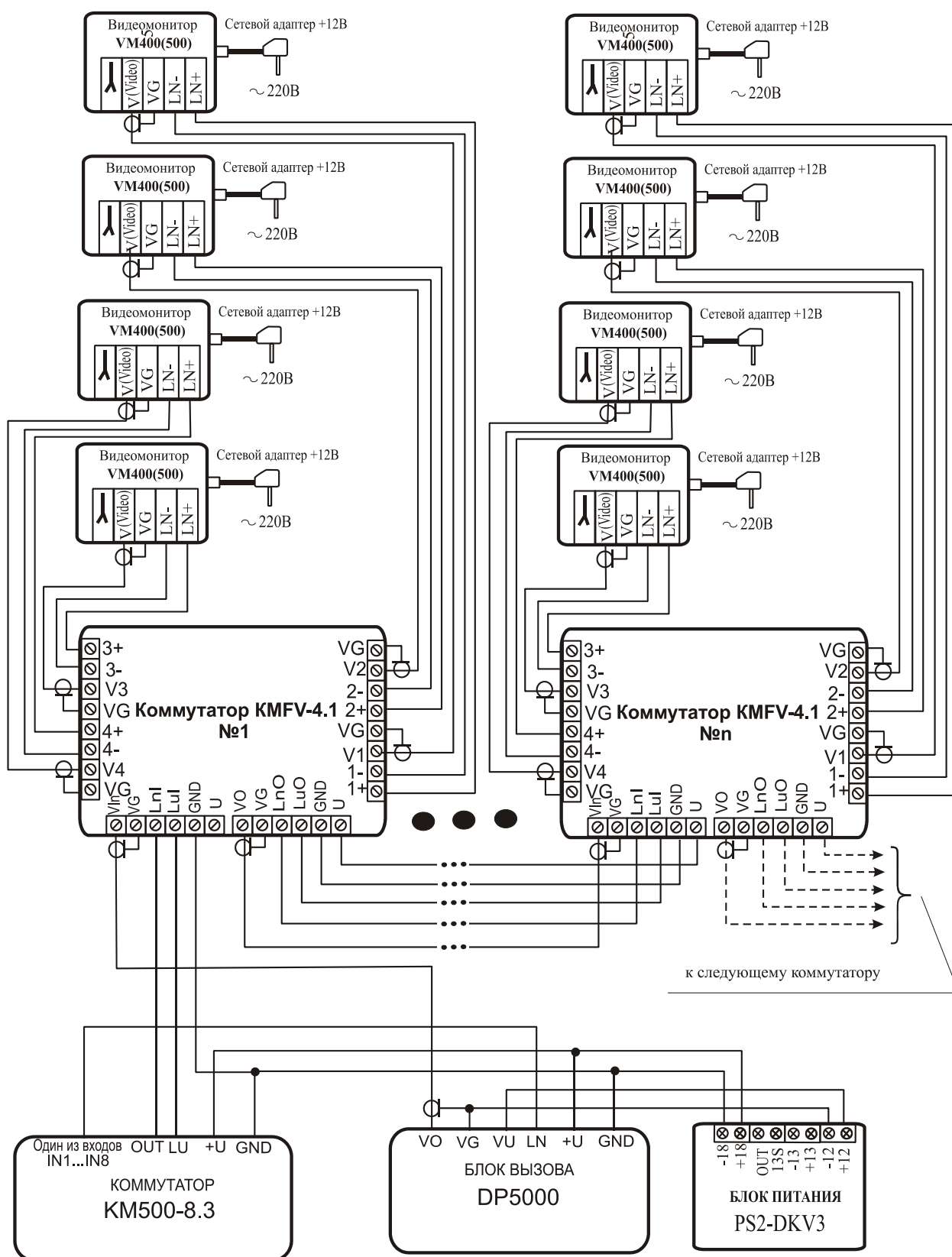
Рис.6 Схема подключения коммутатора этажного КМ- 4.1V в составе сетевого домофонного комплекса ELTIS5000
