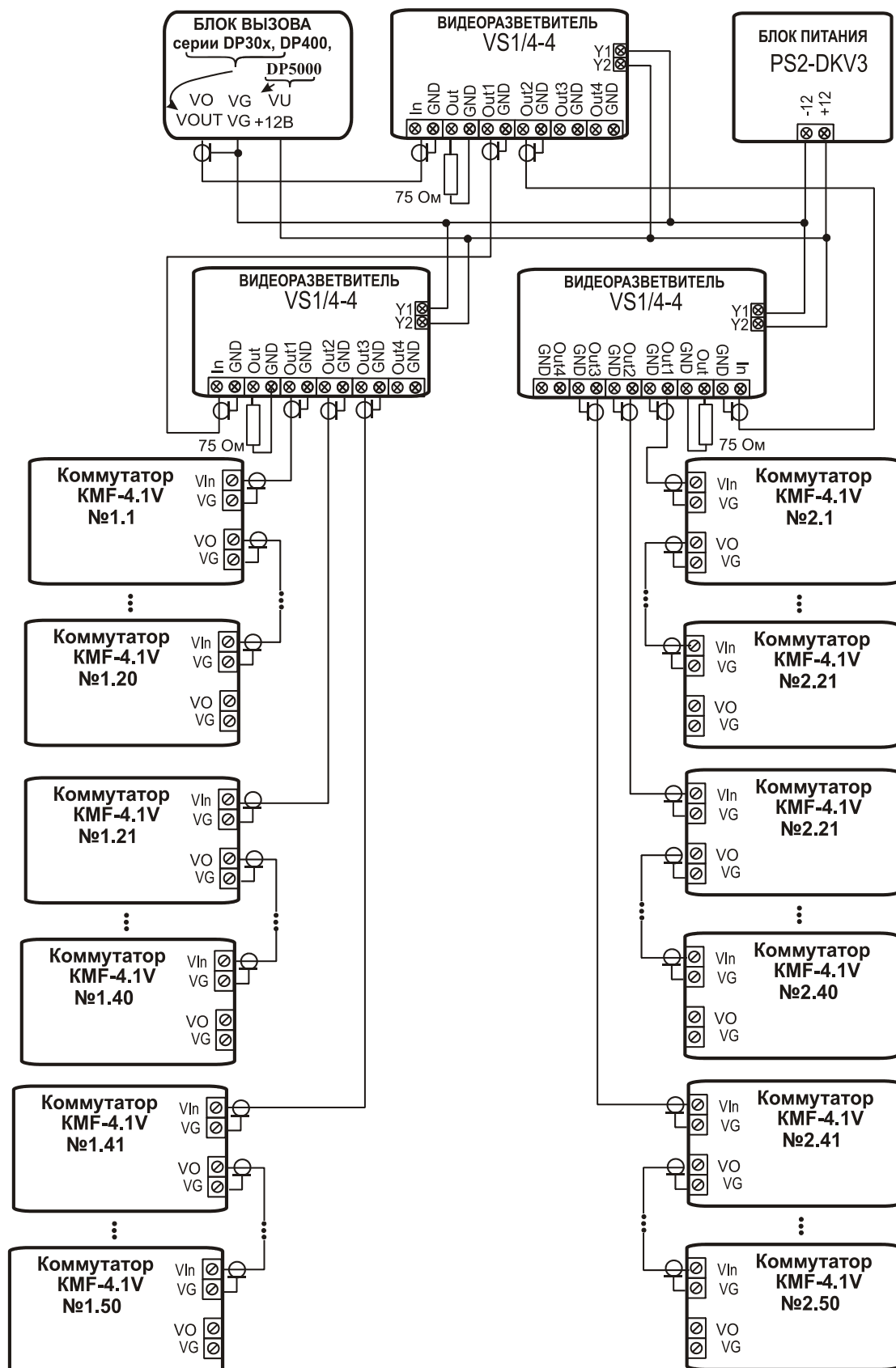
Рис.5 Схема подключения 100 коммутаторов КМ- 4.1V по каналу видео
