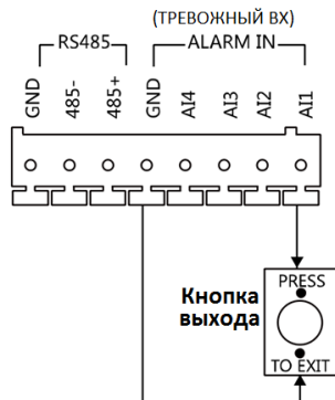
Рисунок 5-22 Подключение кнопки выхода для модели DS-KD6002-VM
