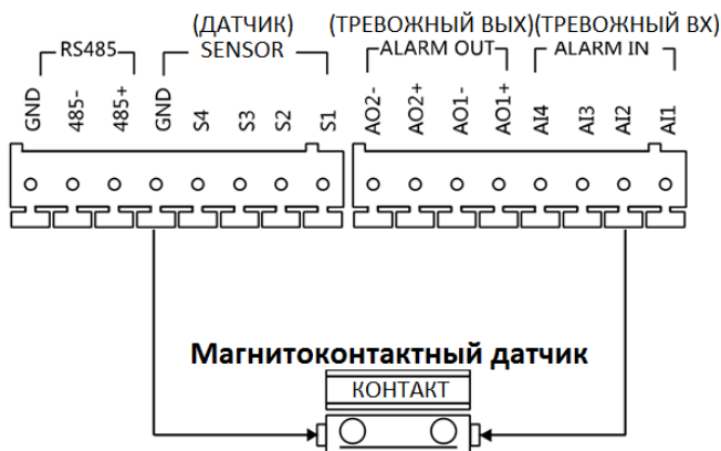
Рисунок 5-17 Подключение магнитоcontactного датчика для моделей DS-KD8102-V/DS-KD8002-VM (1)
