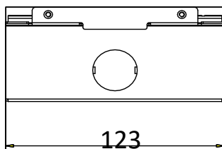
Рисунок 5-1 Вид спереди и сбоку
