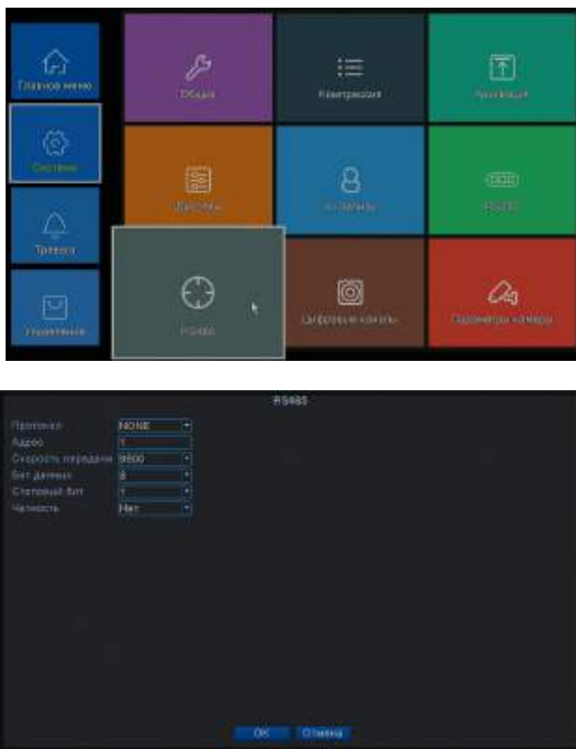
Рисунок 4.33 Конфигурация RS485 устройств в цифровом режиме.
