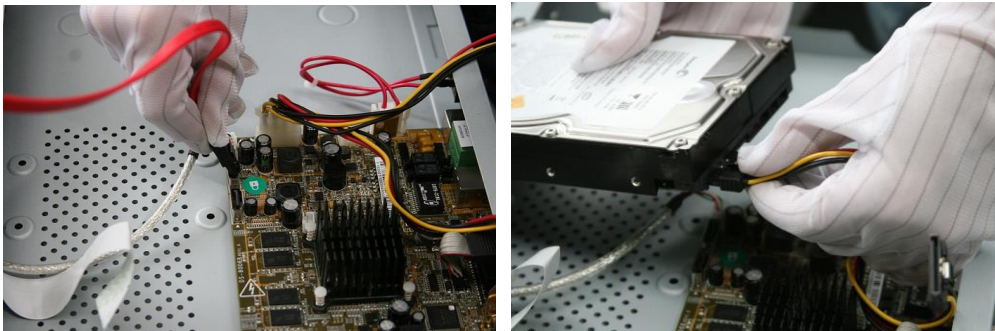
Рисунок 2-2 Подключение кабеля данных
