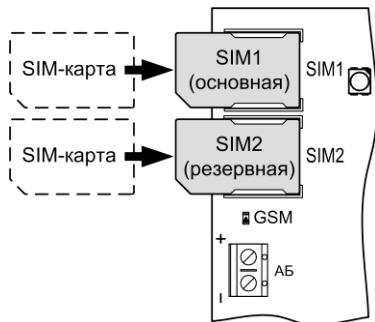
Рис.5 Установка SIM-карт
