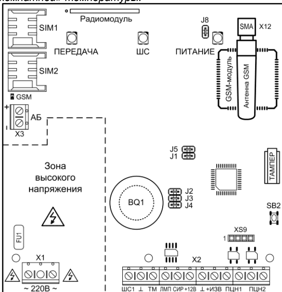
Рис.1 Плата прибора
