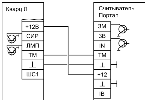
Рис.А3 Схема подключения считывателя «Портал»
