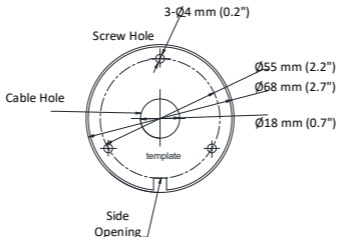
Рисунок 2-2 Шаблон крепления
