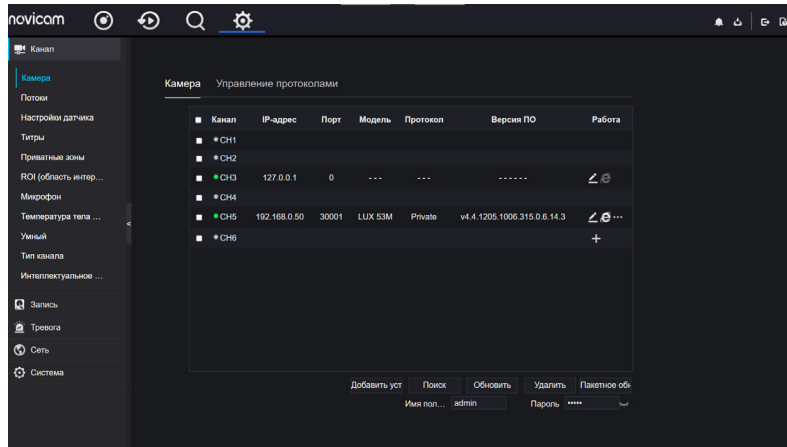
Рис. 42. Интерфейс камеры
