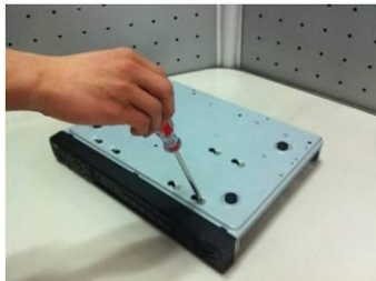
Замацуеце жорсткі дыск на ніжняй панэлі пры дапамозе шруб праз соответствующие адтуліны.
