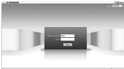
Рис. 5 Окно авторизации.
