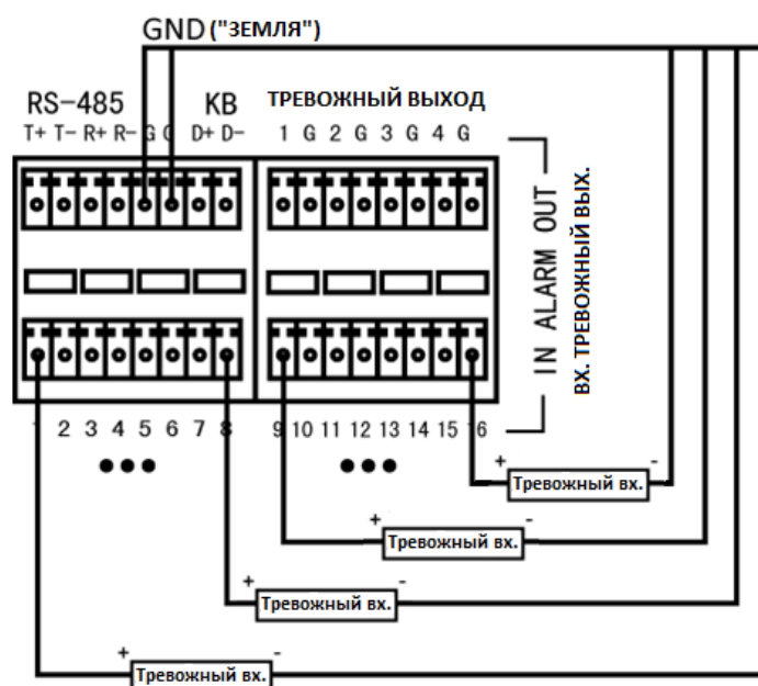
Рисунок 2.10 Подключение тревожного входа
