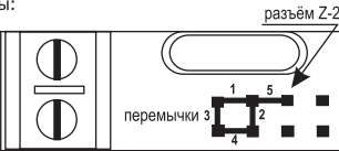
Рис.1 Положения переключки.
