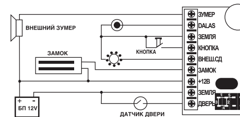
Рис.2 Схема подключения.
