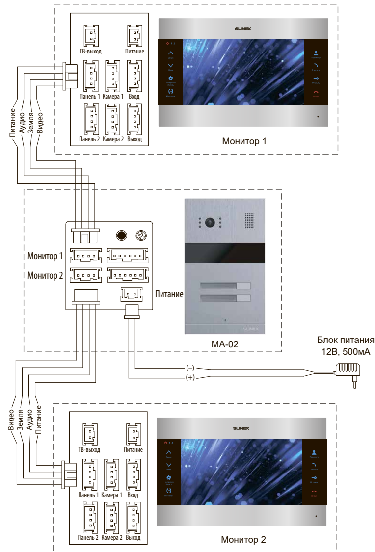
Схема 1. Подключение MA-02 с двумя мониторами.
