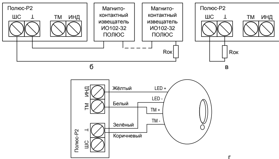
Рис.11б, в, г Схемы подключений к Полус-Р2
