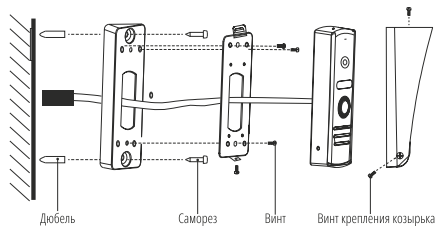
Рис. 9 Установка вызывной панели MASK под углом 30°
