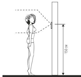
Рис. 4 Рекомендуемая высота установки видеопанели
