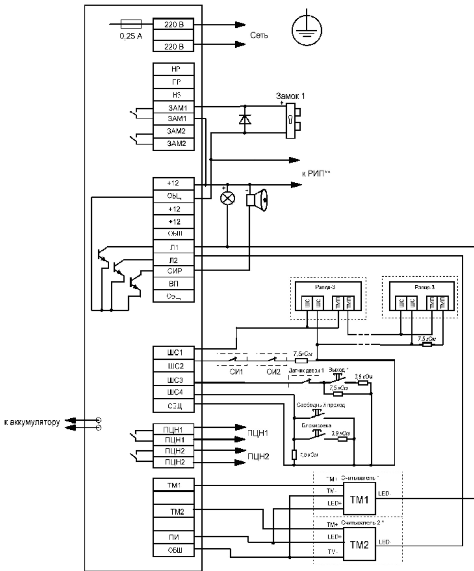
Рисунок 7 – Схема внешних подключений к контроллеру при конфигурации «2ШС+1ТД»
