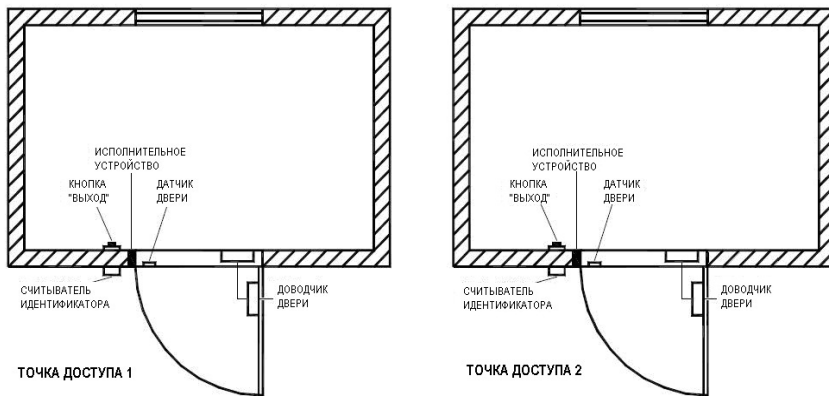
Рисунок 2 – Пункты прохода с контролем входа
