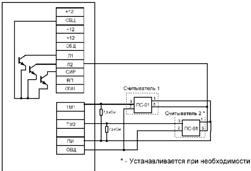
Рисунок 15 – Схема подключения бесконтактных считывателей Proximity карт ПК-01
