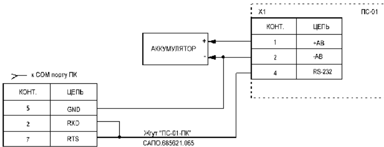
Рисунок 14 – Схема подключения ПК- 01 к компьютеру
