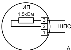
Рис.1 Типовая схема подключения извещателей ИП 101-3А-А3R к ППКОП со знакопостоянным ШПС. Величина резистора Rок определяется в соответствии с техническим описанием ППКОП.
