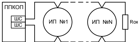
Рис.1 Типовая схема подключения извещателей ИП 101-3А-А3R к ППКОП со знакопостоянным ШПС. Величина резистора Rок определяется в соответствии с техническим описанием ППКОП.
