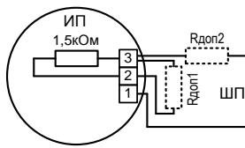
Рис.2 Схемы подключения извещателя к ШПС
