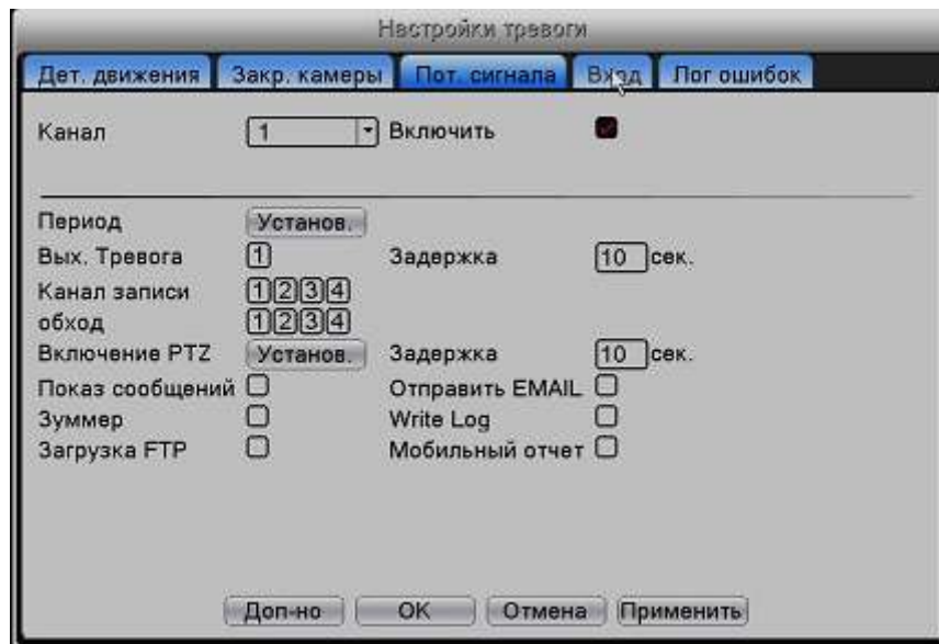
Рис.4-9 Потеря видеосигнала
