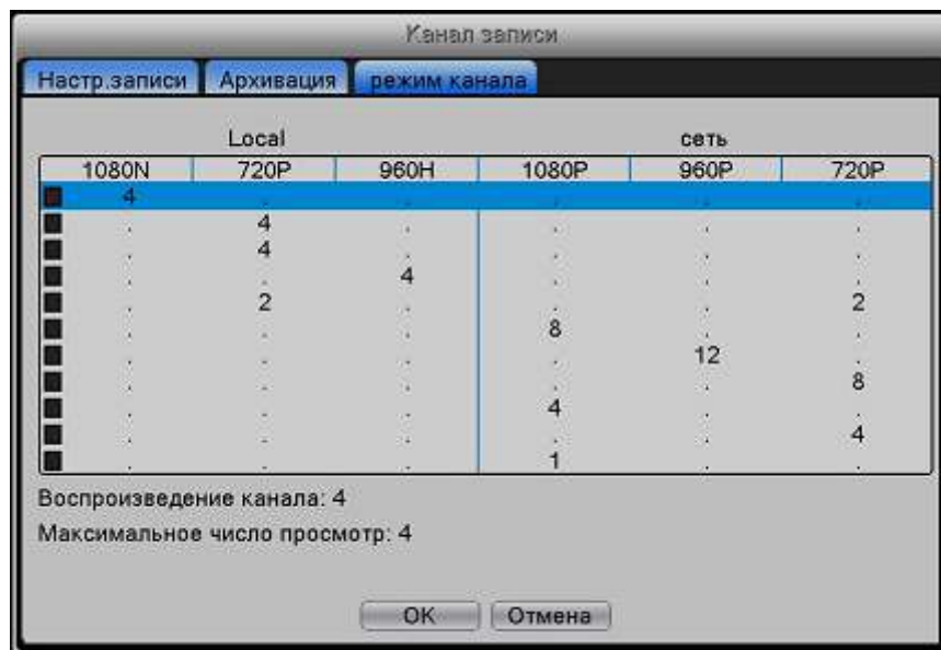
Рис.4-38 Типы канала
