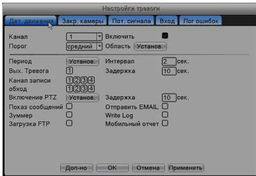
Рис.4-4 Обнаружение движения
