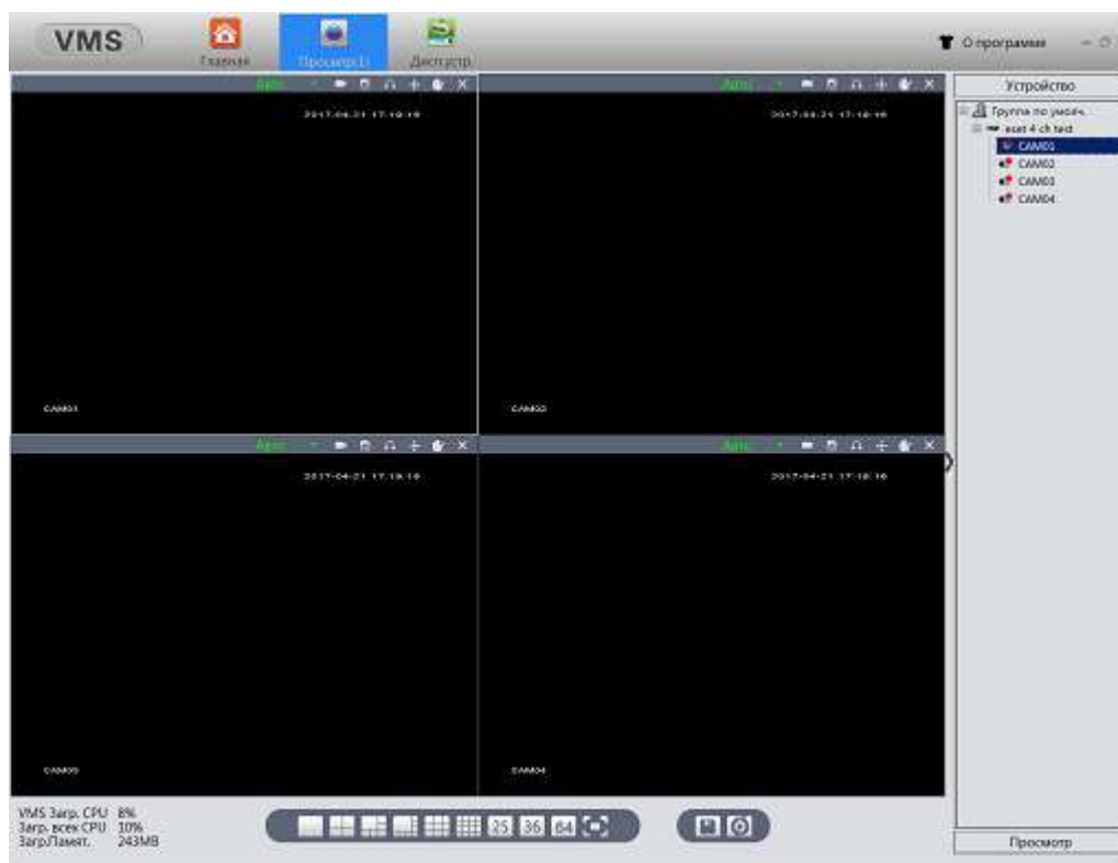
Рис.5-11 Устройство
