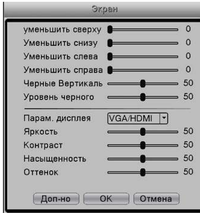
Рис.3-15 Настройки цвета
