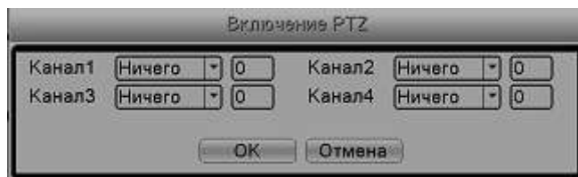
Рис.4-7 Активация PTZ
