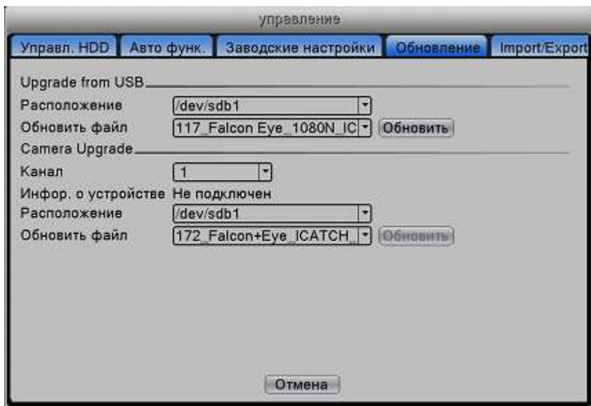
Рис.4-59 Обновление
