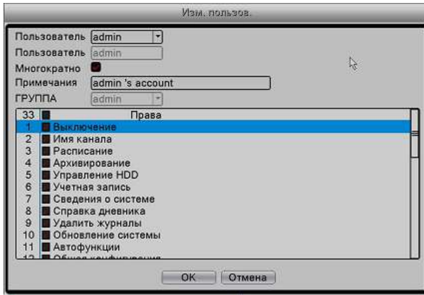
Рис.4-54 Изменение пользователя
