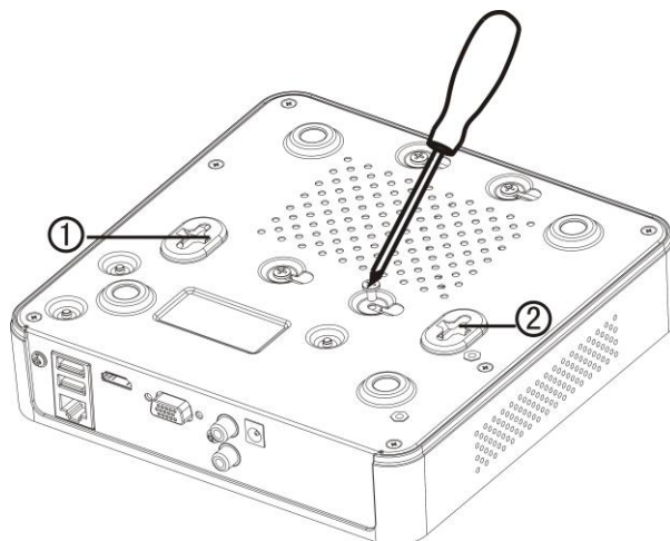
Рисунок 2.2 Установка HDD
