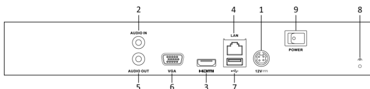
Рисунок 1.4 DS-N3XX
