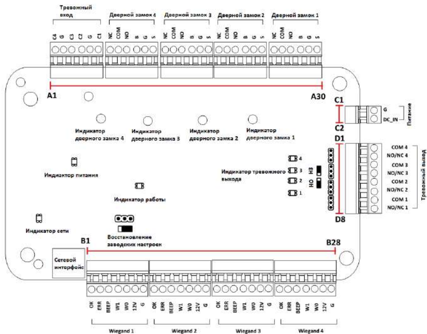
Рисунок 3-3 Клеммы АСТ-С104
