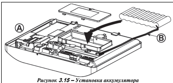
Рисунок 3.15 – Установка аккумулятора
