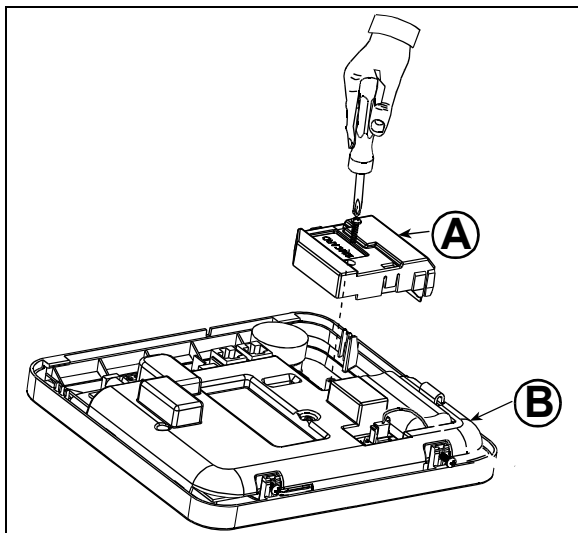
Рисунок 3.5 – Установка GSM модуля
