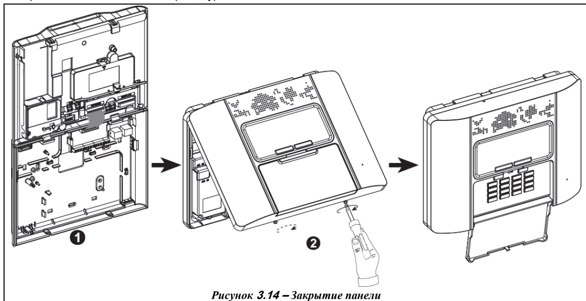
Рисунок 3.14 – Закрытие панели
