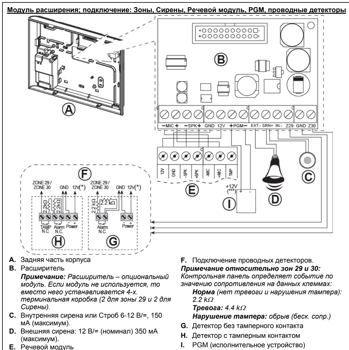
Рисунок 3.23 – Подключение устройств к модулю расширения
