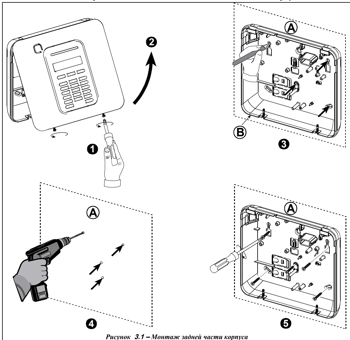
Рисунок 3.1 – Монтаж задней части корпуса
