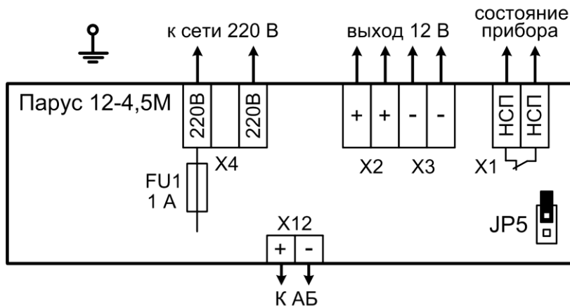
Рис.1 Схема внешних соединений Парус 12-4,5М
