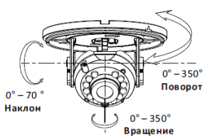
Рисунок 1-11 Настройка угла наблюдения камеры
