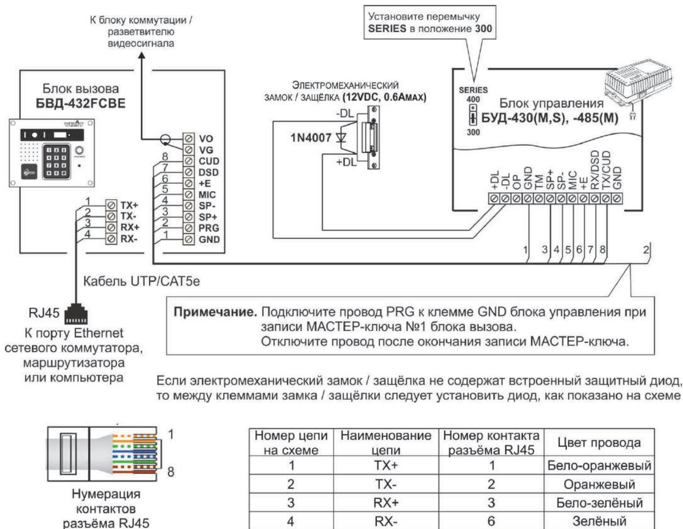
Рисунок 8.3 – Схема соединений блока вызова БВД-432FCBE с блоком управления БУД-430(М,S), -485(М) и электромеханическим замком / защёлкой
