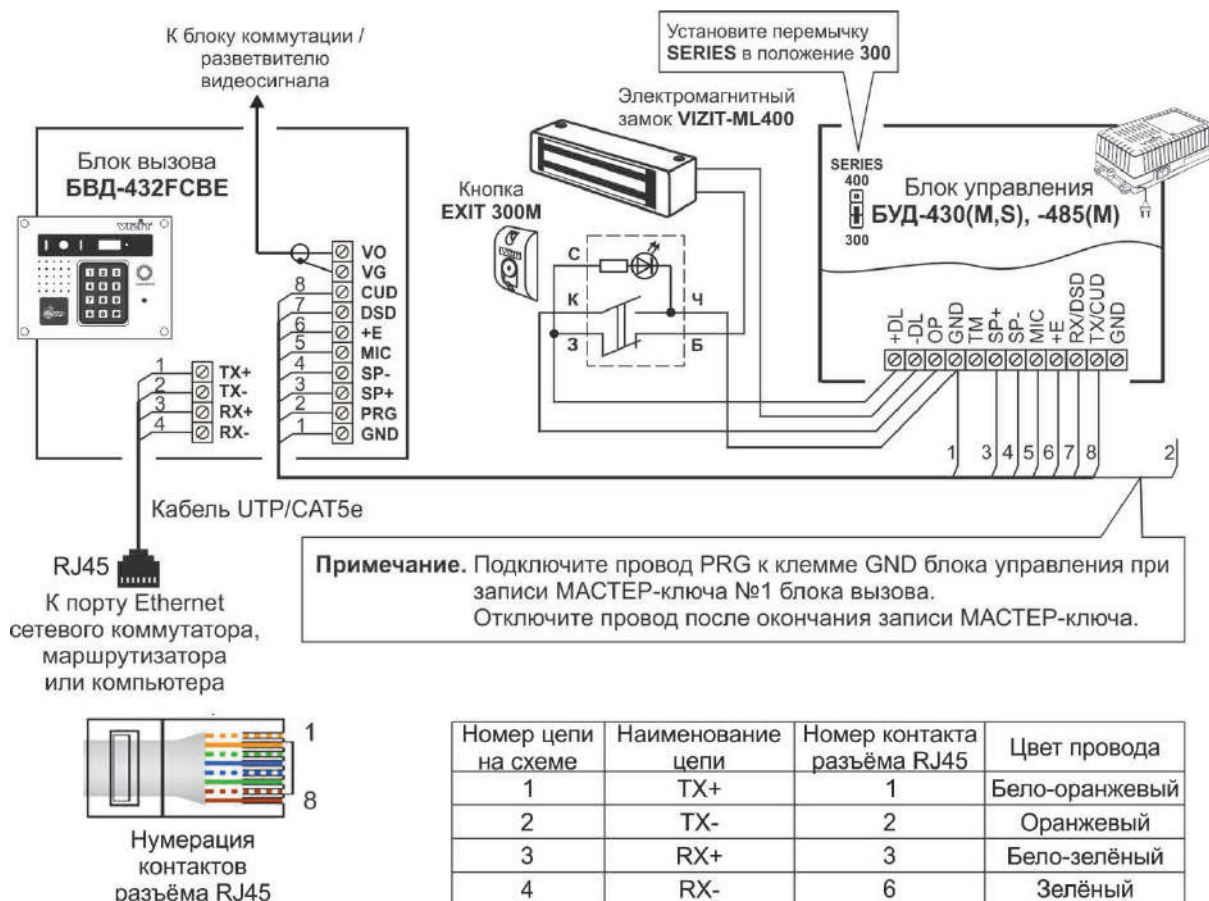
Рисунок 8.1 – Схема соединений блока вызова БВД-432FCBE с блоком управления БУД-430(M,S), -485(M), электромагнитным замком VIZIT-ML400 и кнопкой EXIT 300M
