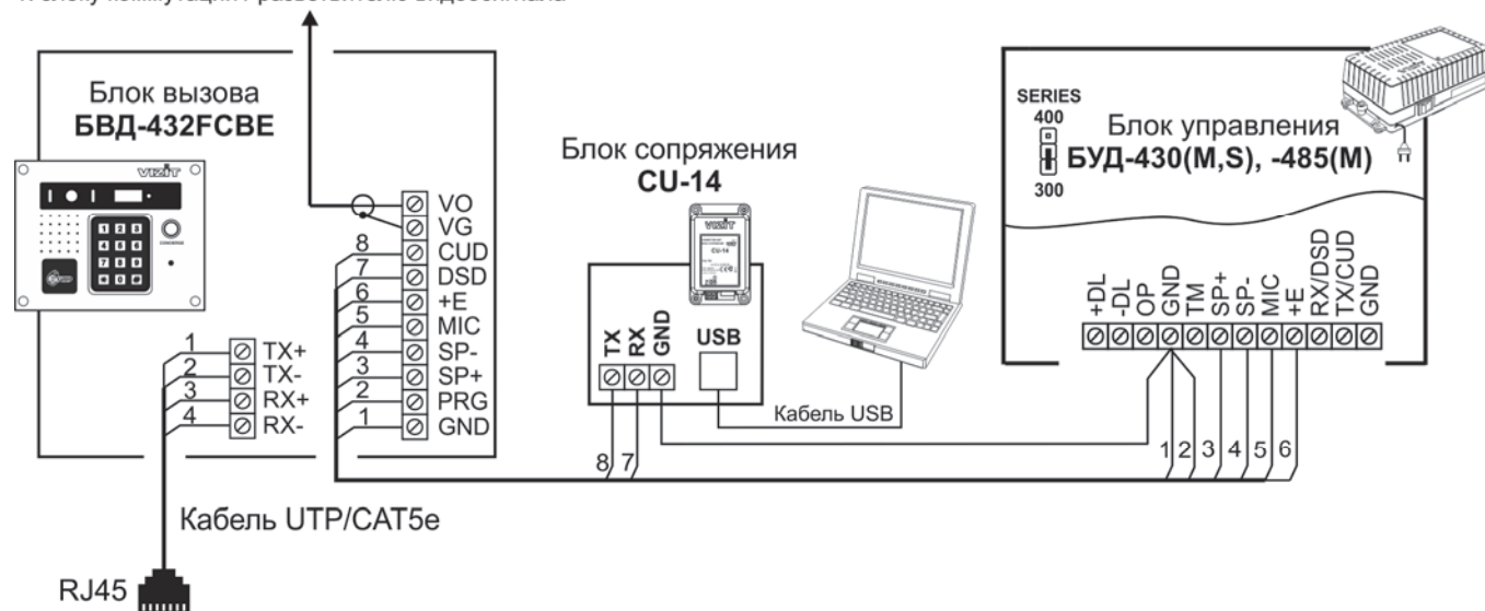
Рисунок 15.1 - Схема соединений блока вызова с блоками управления БУД-430(С, М), -485(М) и блоком сопряжения CU-14
