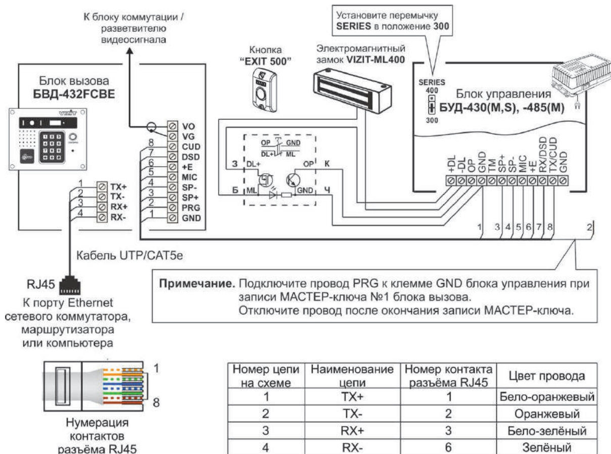
Рисунок 8.2 – Схема соединений блока вызова БВД-432FCBE с блоком управления БУД-430(M,S), -485(M), электромагнитным замком VIZIT-ML400 и кнопкой EXIT 500
