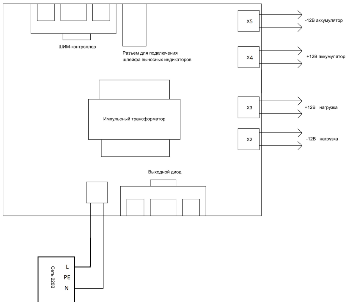
Рис. 1 Схема подключения
